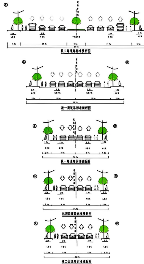
道路断面示意图
